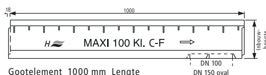
Gooitelement 1000 mm Lengte
