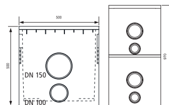
Zandvang/Afvoerput Verhoogde zandvang/afvoerput incl. verzinkte emmer
