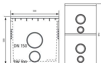
Zandvang/Afvoerput Verhoogde zandvang/ incl. verzinkte emmer afvoerput
