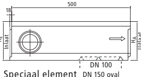
Speciaal element 500 mm
