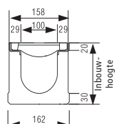
Goothelement 1000 mm bouw lengte
