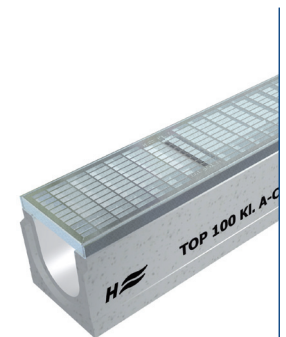
met mazenrooster 30/10
