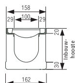
Gotoelement 1000 mm bouwlengte
