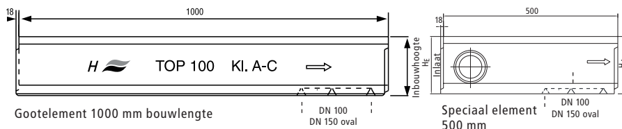
gesloten met Aansluitspie DN 100 Art.Nr.: 1357001110 Art.Nr.: 1357001120
