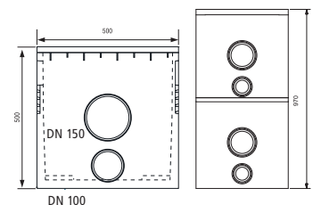
Zandvang/Afvoerput Verhoogde incl. verzinkte emmer zandvang/afvoerput
