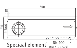
gesloten Art.Nr.: 1357001110 met Aansluitpie DN 100 Art.Nr.: 1357001120
